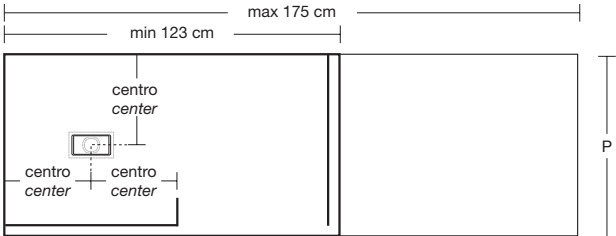
Versione dx - Right version
