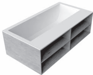
BIBLIO54 H 53,5 P 90 L 170 cm BIBLIO55 H 53,5 P 100 L 180 cm
