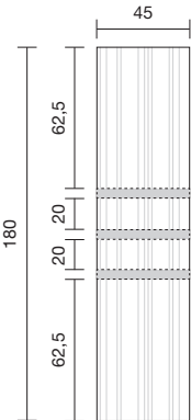
Possibile posizionamento per porta salviette Art. BITBARRA. Possible position of towel holder Art. BITBARRA.
