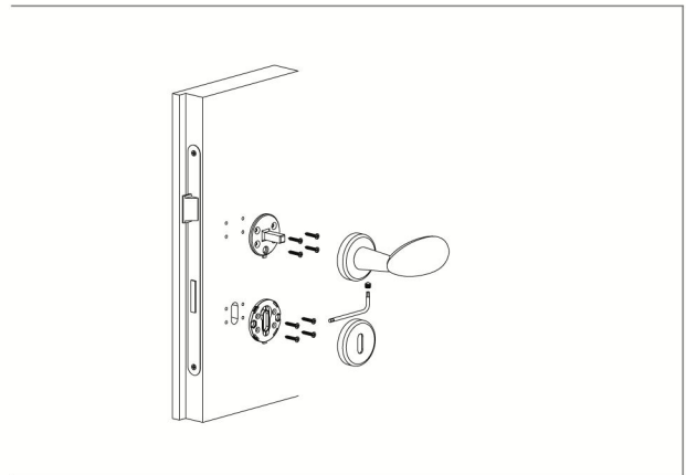
Mezza maniglia fissa con rosetta 911 con quadro 4PxP Fix half-handle on 911 rose with round 4PxP
