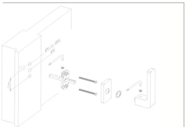
Maniglia per finestra movimento DK regolabile Adjustable drehkipp window system
